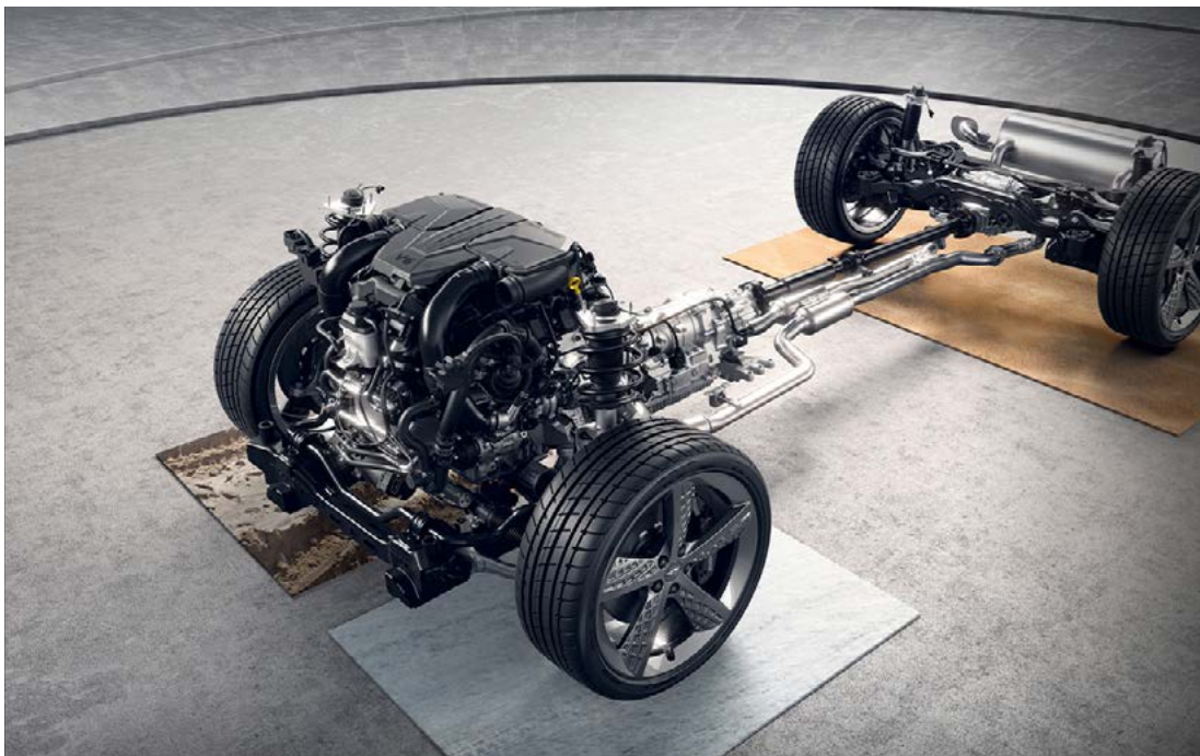
TRACTION INTÉGRALE AVEC SÉLECTION DU MODE DE CONDUITE
