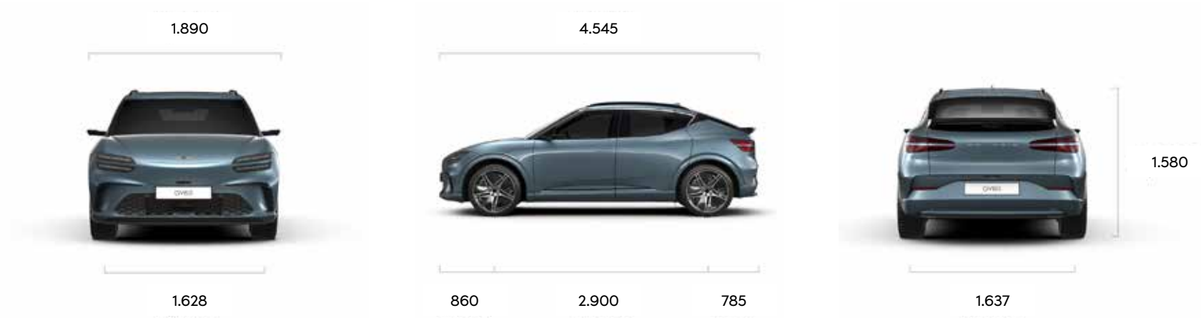
AFMETINGEN (MM), INCL. DAKRAILS
